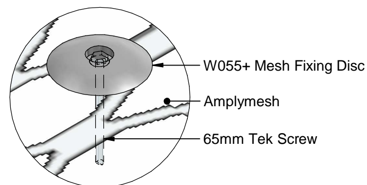
DETAIL 1 1:2
